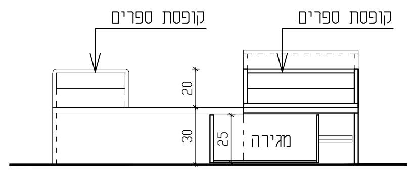
חתך 2-2
